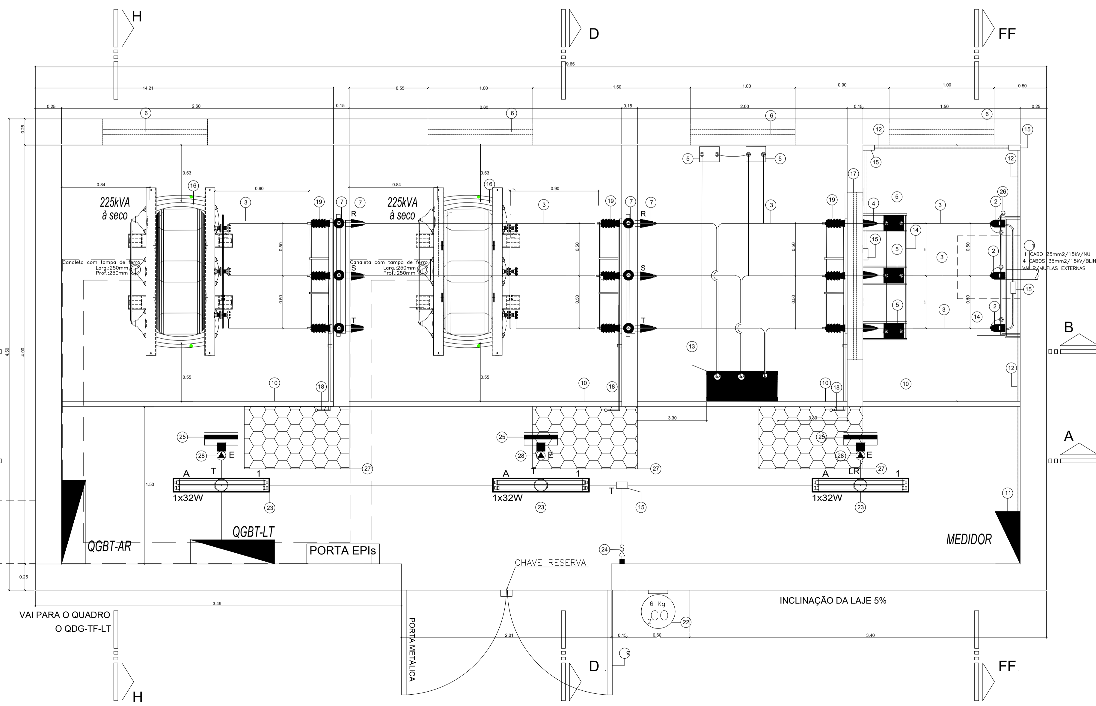
Planta Baixa da Subestação escala 1/20
