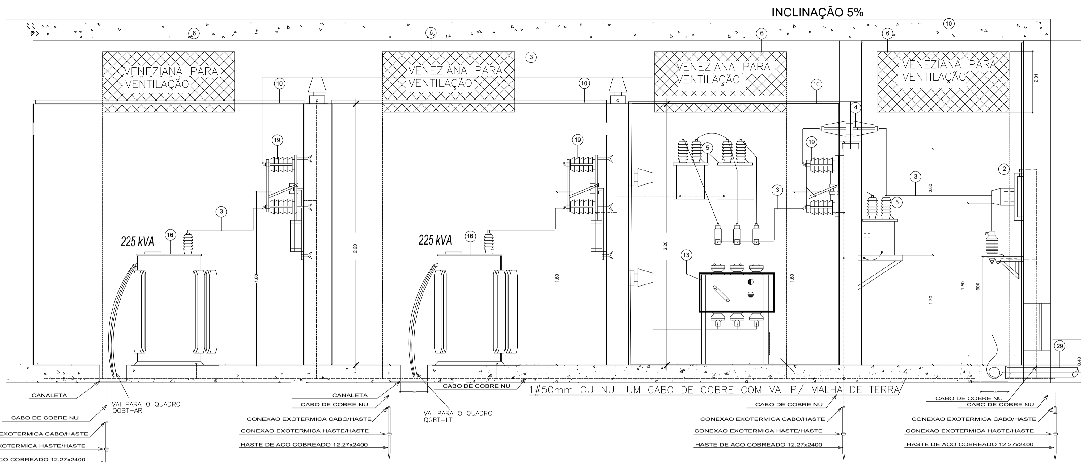
CORTE B-B' - Subestação escala 1/20
