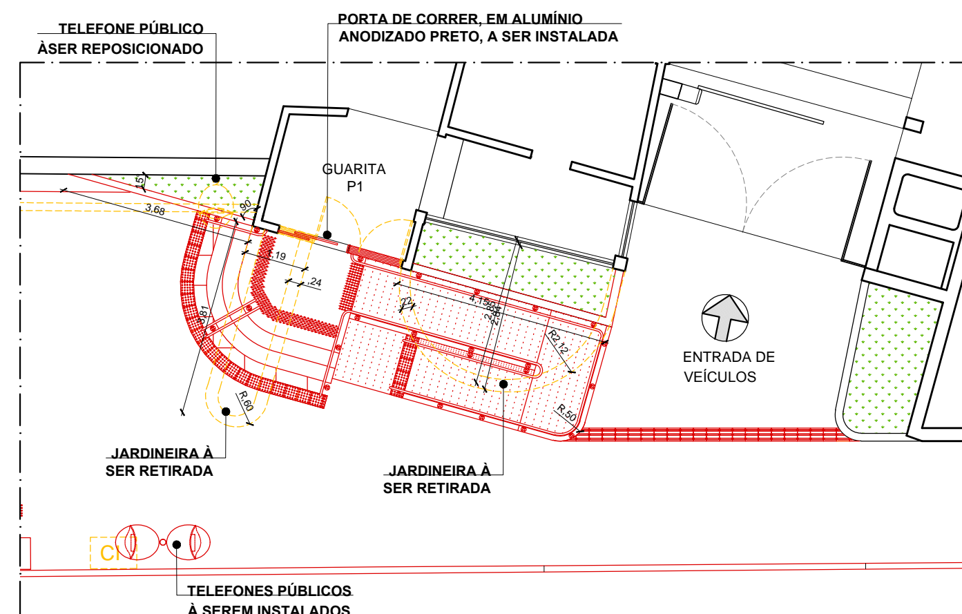
01 PLANTA-BAIXA DE REFORMA/CONSTRUÇÃO - ENTRADA VEÍCULOS - GUARITA P1 ESCALA 1/100
