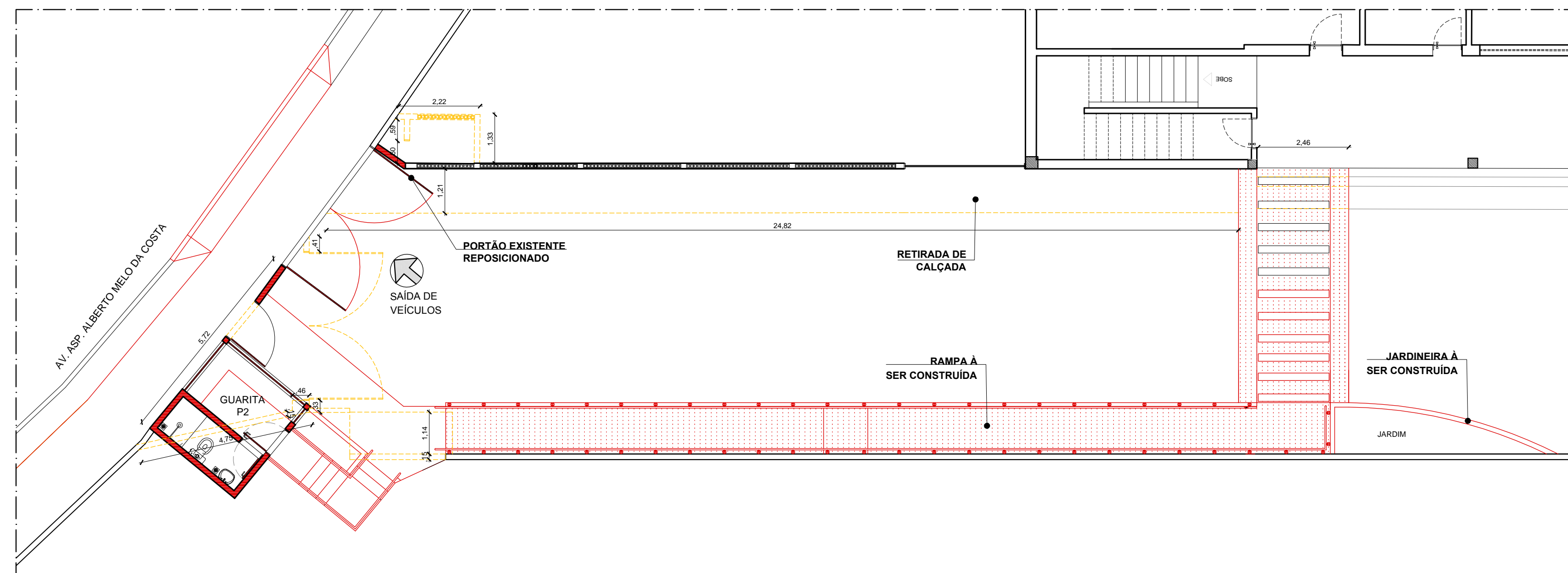
02 PLANTA-BAIXA DE REFORMA/CONSTRUÇÃO - SAÍDA DE VEÍCULOS - GUARITA P2 ESCALA 1/100
