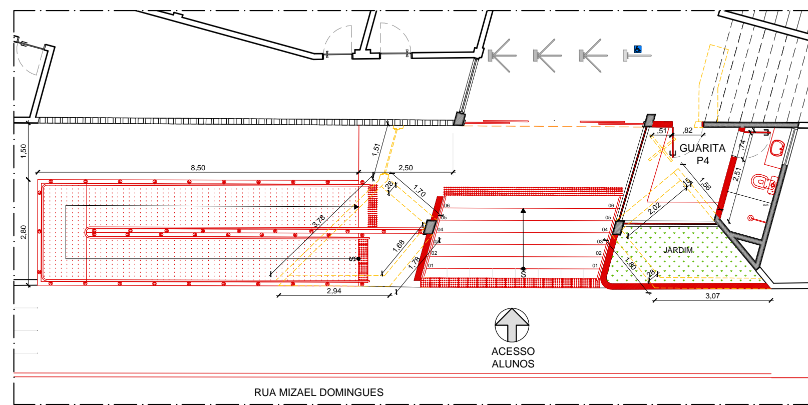
04 PLANTA-BAIXA DE REFORMA/CONSTRUÇÃO - GUARITA P4 ESCALA 1/100
