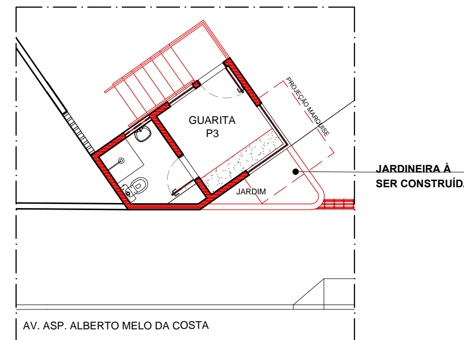
03 PLANTA-BAIXA DE REFORMA/CONSTRUÇÃO - GUARITA P3 ESCALA 1/100
