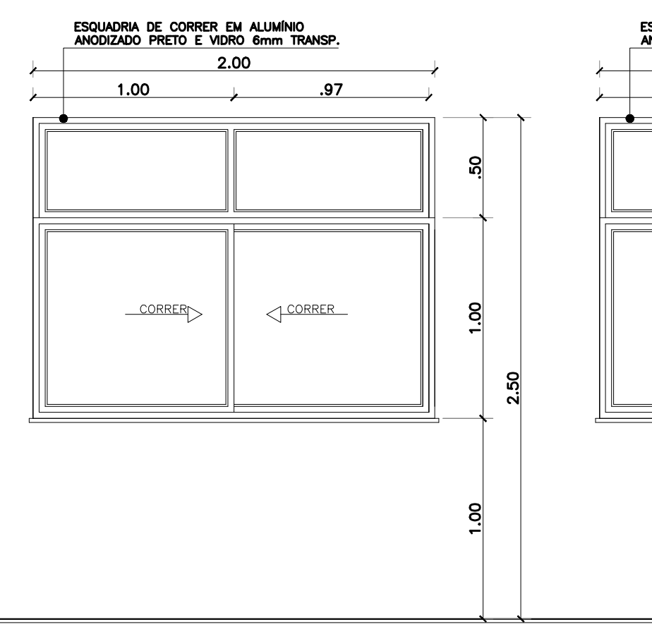
27 ESQUADRIA JA3 ESC. - 1/50
