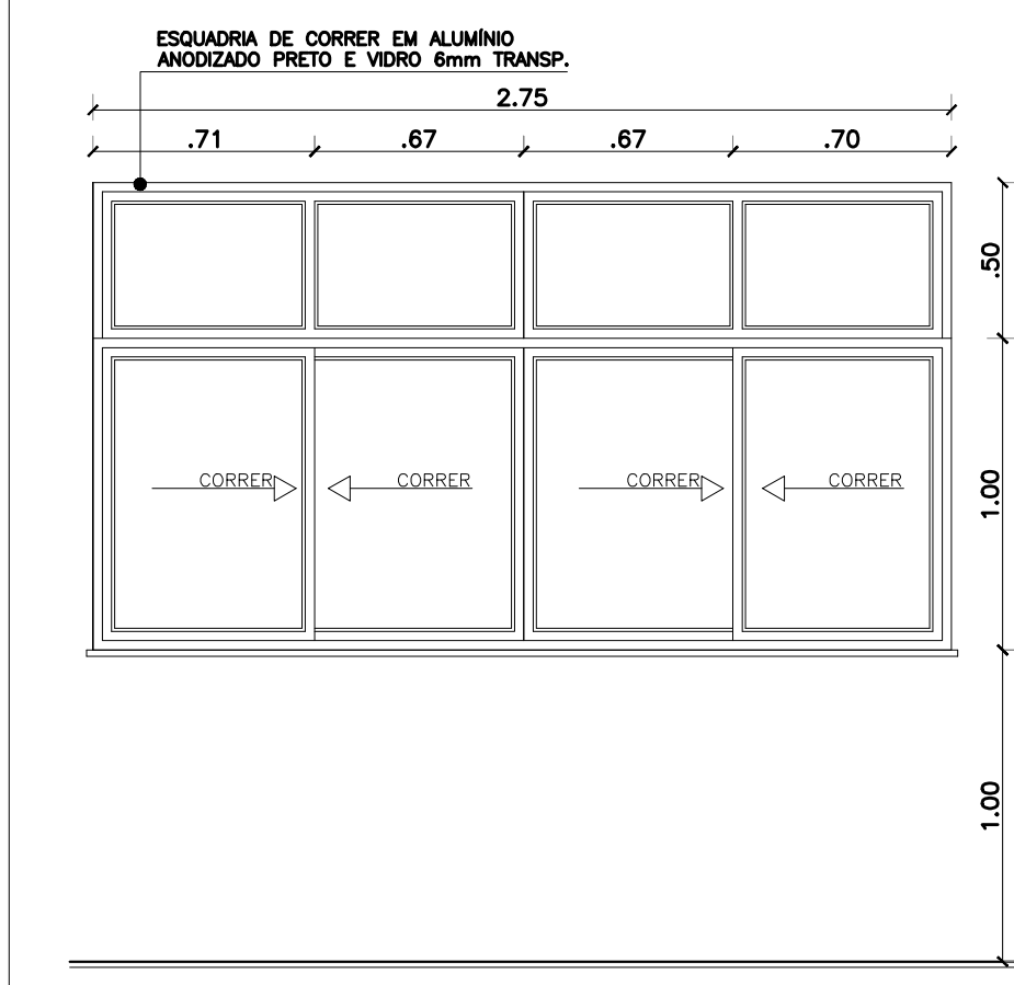
25 ESQUADRIA JA1 ESC. - 1/50
