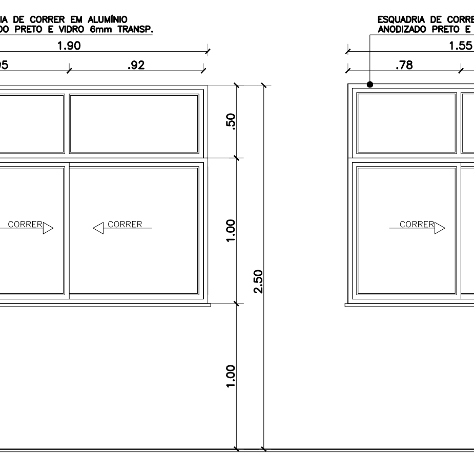
28 ESQUADRIA JA4 ESC. - 1/50
