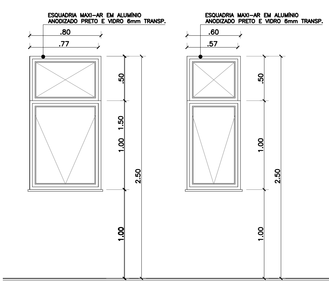
30 ESQUADRIA JA6 ESC. - 1/50
