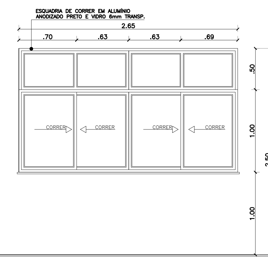
26 ESQUADRIA JA2 ESC. - 1/50
