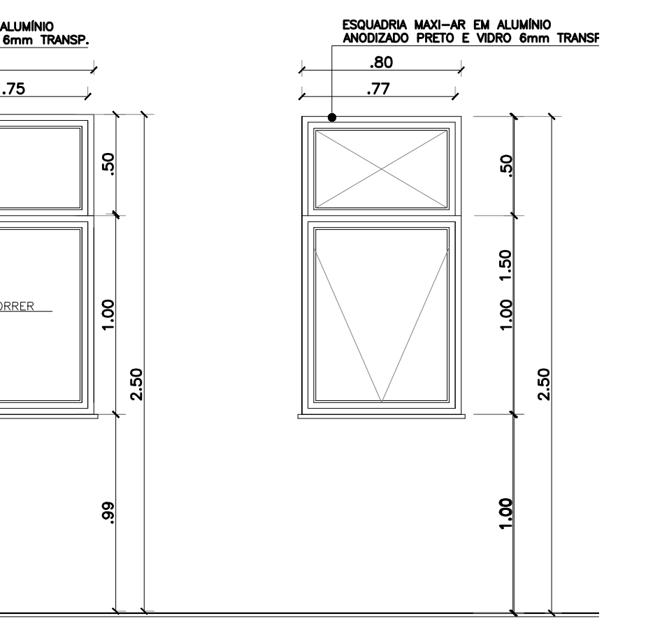
29 ESQUADRIA JA5 ESC. - 1/50
