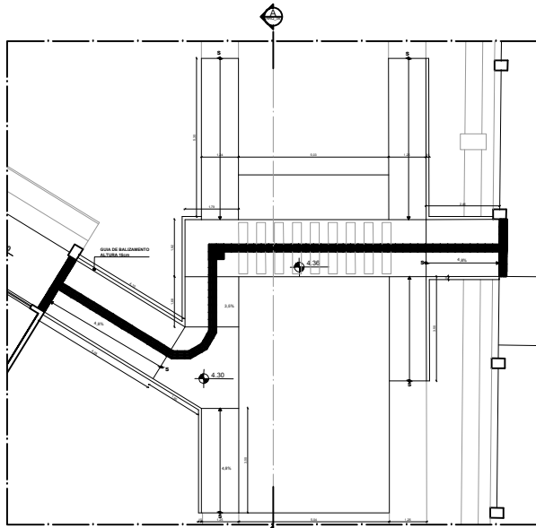
01 DETALHE D1 ESCALA 1:50
