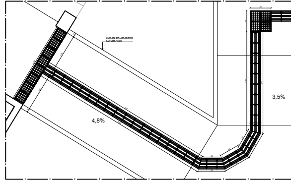
02 IMPLANTAÇÃO D1 ESCALA 1:50
