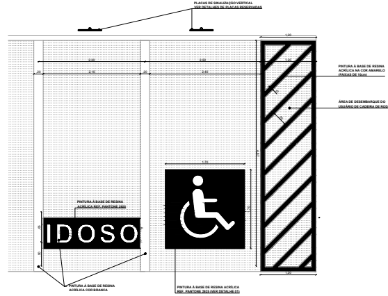
06 DETALHE VAGAS RESERVADAS ESCALA 1:50
