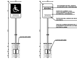
11 DET. PLACAS RESERVADAS ESCALA 1:50
