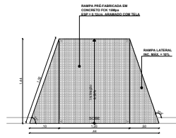
04 DET. RAMPA - MODELO 02 ESCALA 1:50
