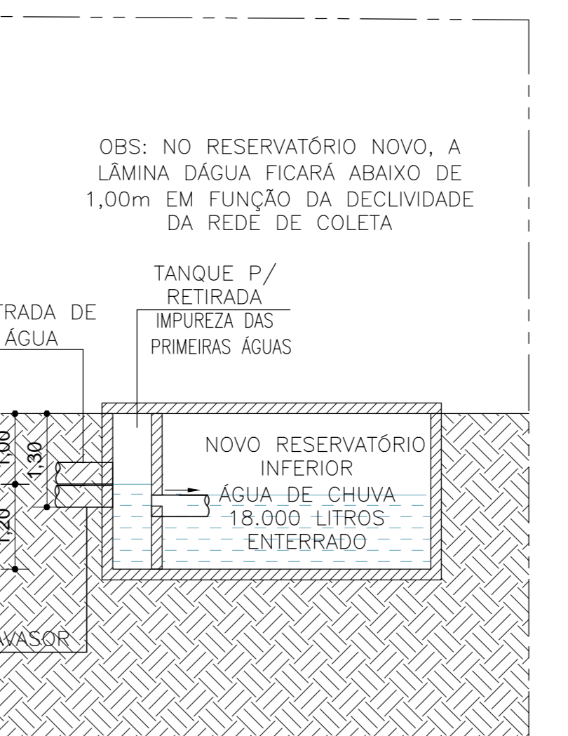
CORTE BB - ESQUEMÁTICO
