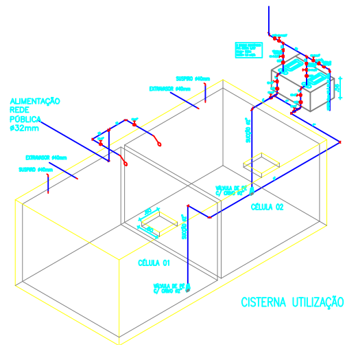
DETALHE ISOMÉTRICO CISTERNA UTILIZAÇÃO ESCALA: 1/10
