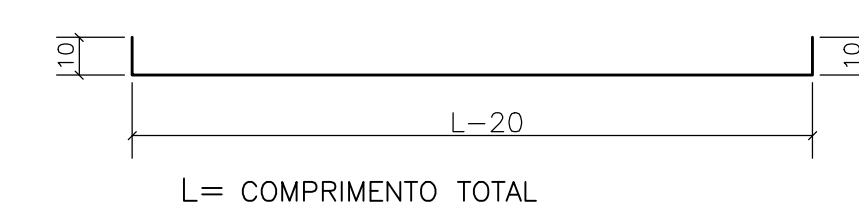
DET. PADRÃO DA ARMADURA POSITIVA DAS NERVURAS
