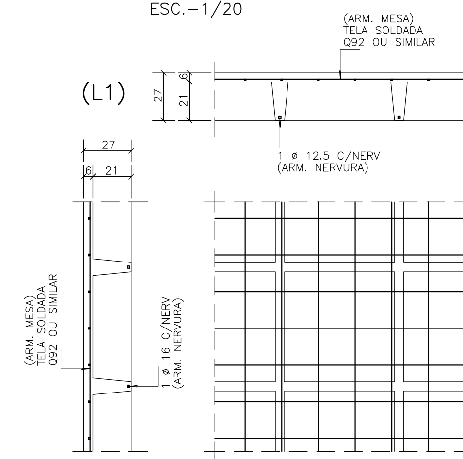
DET. PADRÃO DA LAJES NERVURADAS. ESC.-1/20
