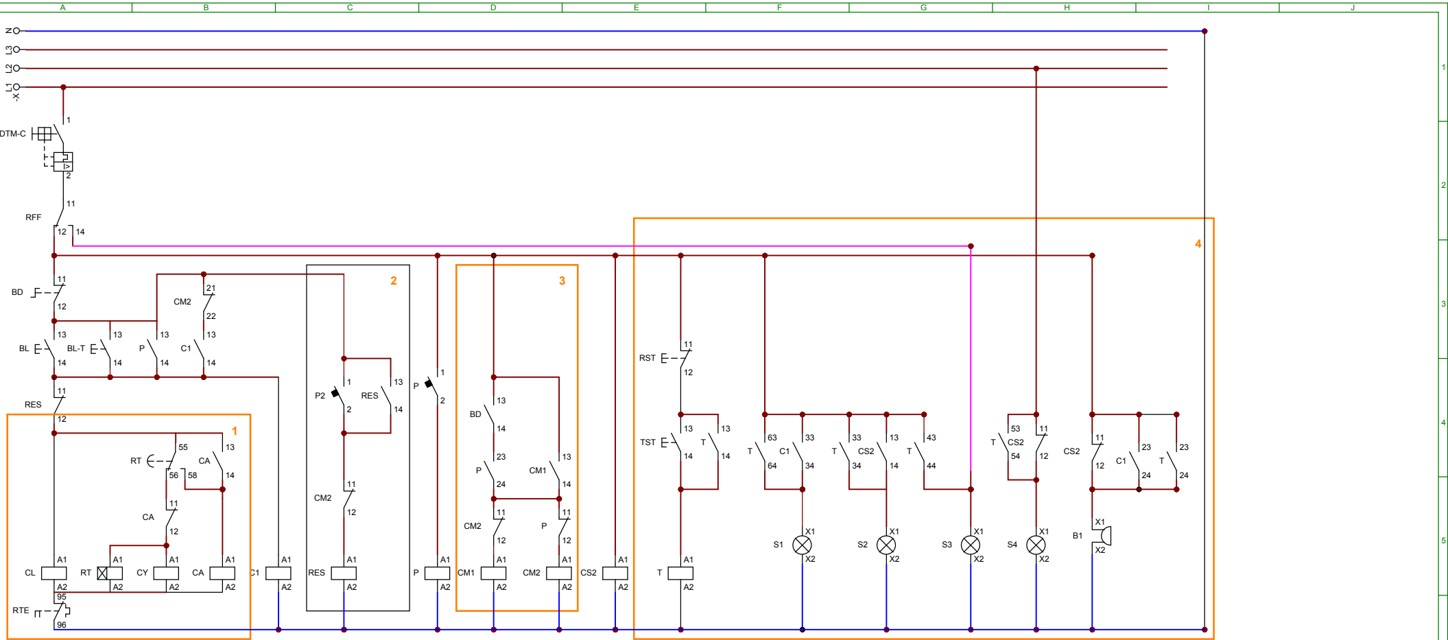
Partida da Motobomba
