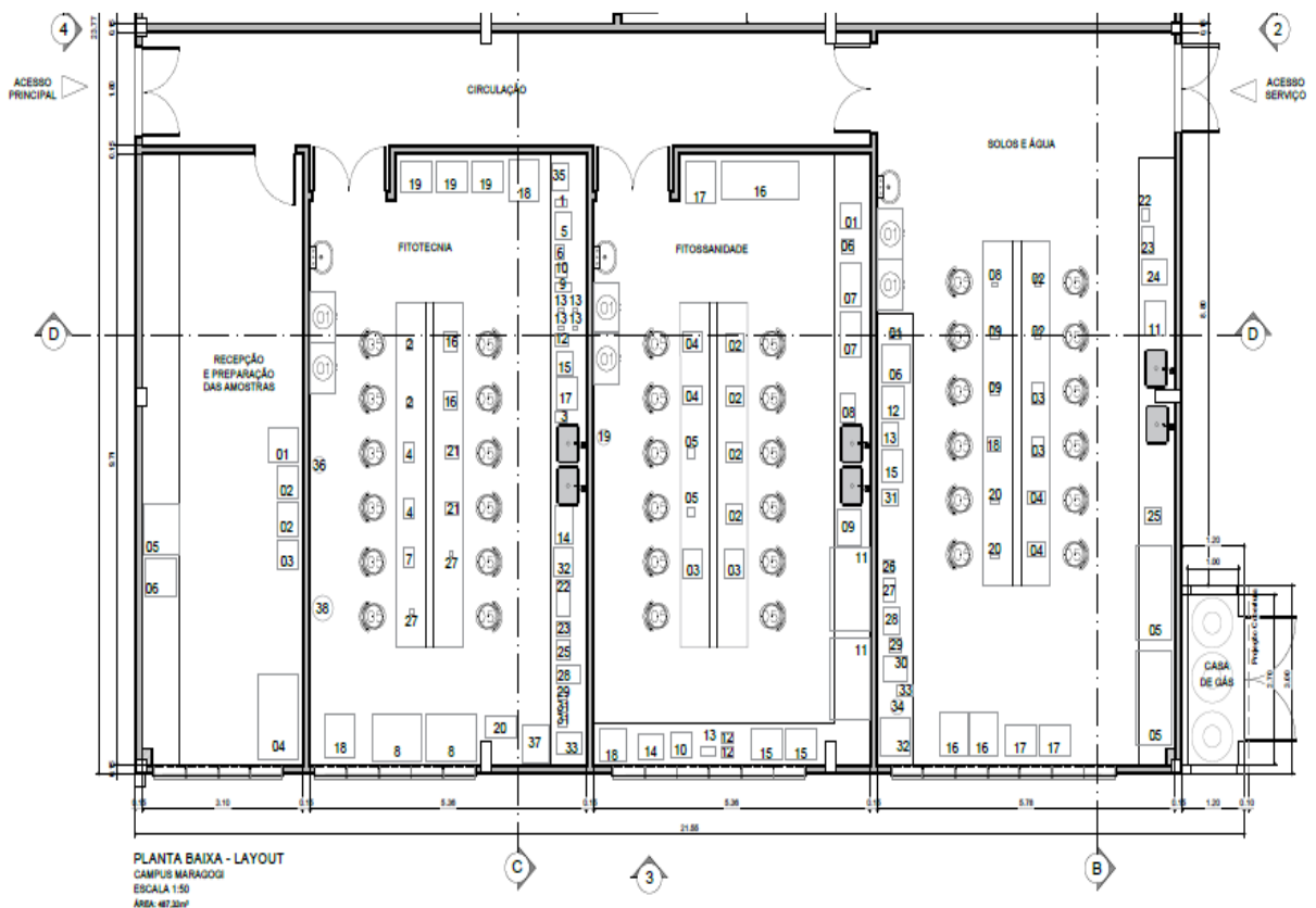
Figura 2 – Planta do Complexo de Laboratórios Especiais de Agroecologia
